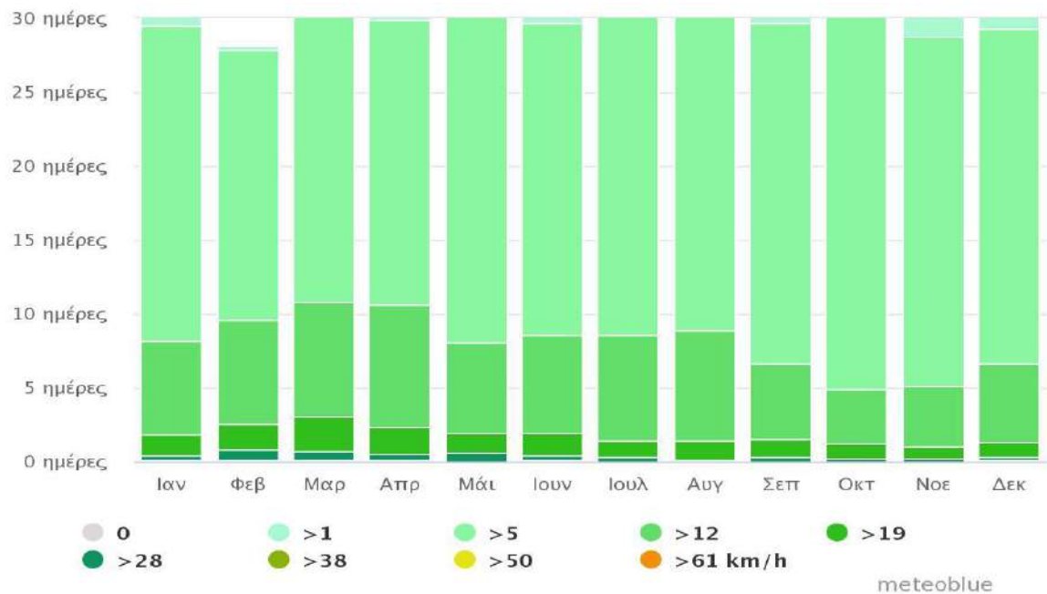
Διάγραμμα: Ταχύτητα ανέμου με βάση στατιστικά στοιχεία των τελευταίων 30 ετών (Πηγή : meteoblue.com)
