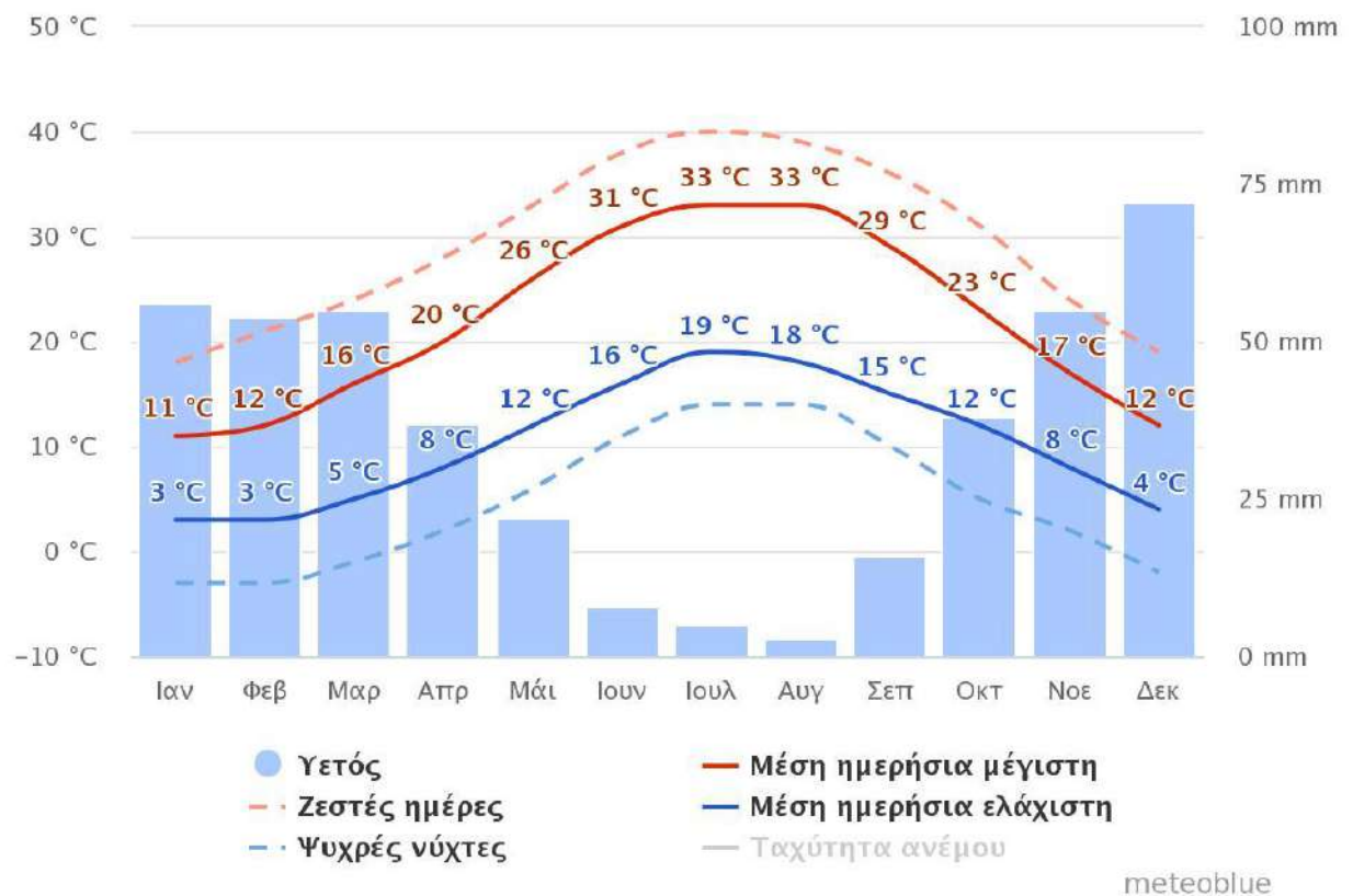
Διάγραμμα: Μέσος όρος θερμοκρασιών και βροχοπτώσεων με βάση στατιστικά στοιχεία των τελευταίων 30 ετών (Πηγή : meteoblue.com)
